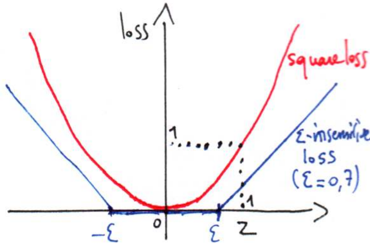
FIGURE 8.7 – Coûts quadratique et \epsilon -insensitive.
