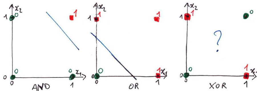
FIGURE 9.3 – Les calculs de AND, OR, ou XOR peuvent être vus comme des problèmes de classification binaire. Les opérateurs logiques AND et OR sont calculés par un classifieur linéaire (donc un perceptron), contrairement à l'opérateur XOR.
