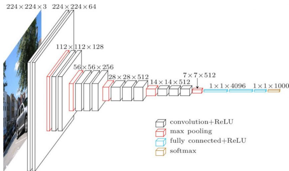
FIGURE 10.5 – Un exemple de réseau convolutif profond : VGG16 (K. Simonyan and A. Zisserman, 2014). L'entrée est constitué de 224 \times 224 \times 3 = 150528 neurones, ce qui correspond à une image couleur (trois canaux) de 224 \times 224 pixels. Le premier bloc de convolutions est constitué de 64 filtres indépendants de support de taille 3 \times 3 \times 3 , chacun étant suivi d'une activation ReLU. Un second bloc réalise la même opération. Ensuite, un seul pixel sur deux est gardé dans le pooling. Les blocs de convolution et de pooling se succèdent jusqu'à atteindre un réseau complètement connecté classique constitué de deux couches de 4096 neurones, une couche de 1000 neurones, puis une couche SoftMax de 1000 neurones (il s'agit d'un problème de classification à 1000 classes). Ce réseau est gouverné par 138 millions de paramètres. Par exemple les connexions entre l'entrée et la première couche de convolution nécessitent (3 \times 3 \times 3 + 1) \times 64 = 1792 paramètres (64 filtres 3 \times 3 sur les 3 composantes RVB, et un biais par filtre), et entre la première et la deuxième couche de convolution (3 \times 3 \times 64 + 1) \times 64 = 36928 paramètres. Source de l'illustration : https://neurohive.io/en/popular-networks/vgg16/ où sont fournis les détails de l'architecture.
