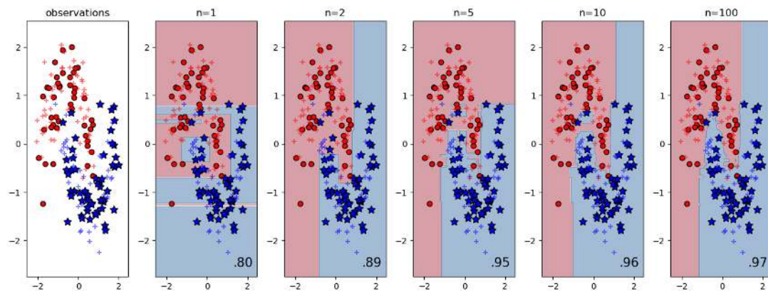
FIGURE 7.4 – Classification de données bidimensionnelles à l'aide de la fonction RandomForestClassifier de scikit-learn, pour différents nombres n d'arbres dans la forêt. Les arbres aléatoires sont construits sur une caractéristique ( m = 1 ). Les observations sont séparées en deux classes, des observations tests (croix en transparence) permettent de calculer un taux de classifications correctes, indiqué en bas à droite. On voit que plus la forêt contient d'arbres, plus la frontière de classification est complexe.
