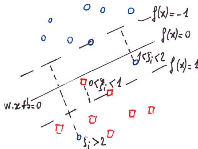
FIGURE 8.2 – SVM : marge souple et variables d'écart. Notons les valeurs prises par \xi_i selon la position de l'observation \mathbf{x}_i par rapport à la droite de séparation. Ici, f(\mathbf{x}) = \mathbf{w} \cdot \mathbf{x} + b .
