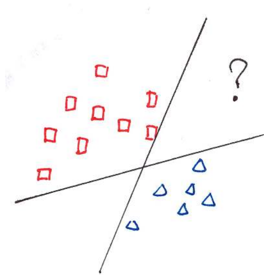
FIGURE 9.2 – Perceptron : ambiguïté de l'hyperplan séparateur obtenu. Selon l'hyperplan retenu, une observation non étiquetée sera associée à une classe ou à l'autre.
