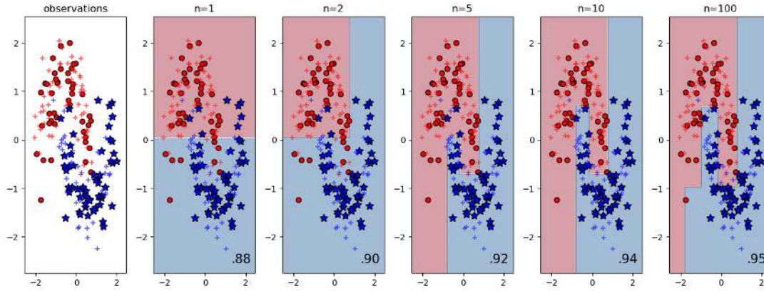
FIGURE 7.6 – Classification de données bidimensionnelles à l'aide de la fonction AdaBoostClassifier de scikit-learn, pour différents nombres n de classifieurs faibles. Les classifieurs faibles sont des troncs de classification. Les observations sont séparées en deux classes, des observations tests (croix en transparence) permettent de calculer un taux de classifications correctes, indiqué en bas à droite. Là aussi, plus le nombre de troncs est grands, plus la frontière de classification est complexe.
