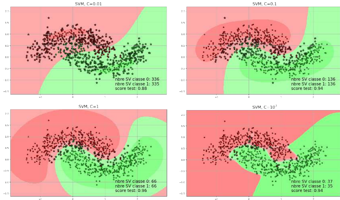
FIGURE 8.5 – Exemples de classification obtenues dans un problème biclasse (classe 0 en rouge et classe 1 en vert) pour quatre valeurs de C . Les vecteurs supports sont marqués d'une étoile. On indique à chaque fois le nombre de vecteurs supports dans chaque classe ainsi que le score de classification obtenues sur des observations test (non représentées) qui n'ont pas servi à l'apprentissage. La marge apparaît en clair. Cette expérience illustre qu'un C petit induit un sous-apprentissage, et un C trop grand un sur-apprentissage. Figure à voir en couleur.
