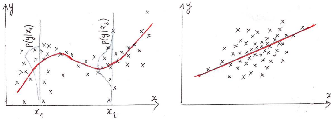
FIGURE 4.1 – Régression pour un coût quadratique. Dans ces exemples, on souhaite prédire y \in \mathbb{R} en fonction de l'observation x \in \mathbb{R} . L'estimateur optimal est représenté en trait plein et est donné en chaque x par : h(x) = \int y p(y|x) dy = E(Y|X = x) . À gauche : situation générale dans laquelle la forme de la densité p(y|x) varie selon x . À droite : lorsque (X, Y) est un vecteur gaussien, h est un estimateur linéaire.
