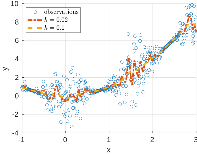
FIGURE 4.2 – Régression à noyau de Nadaraya-Watson. Le noyau est ici une fonction gaussienne d'écart-type h . On voit l'effet régularisateur du paramètre h , qui gouverne la taille du noyau.
