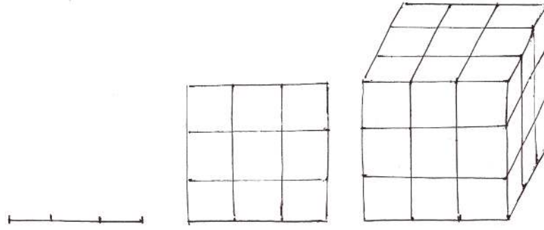
FIGURE 2.1 – Évolution du nombre de cubes de côté de longueur 1/n nécessaires pour remplir le cube unité dans \mathbb{R}^d (ici, n = 3 ).
