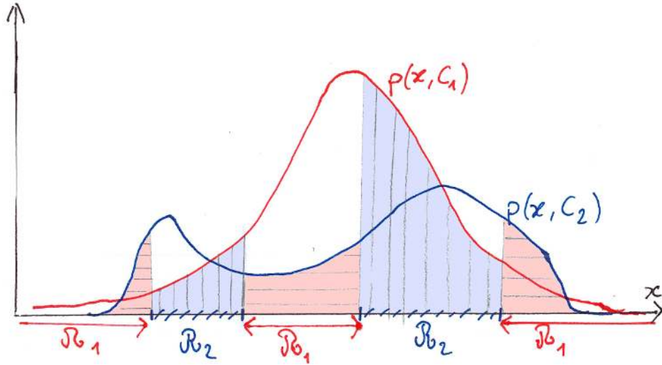
FIGURE 4.3 – Minimisation du risque de prédiction. Nous représentons les densités p(\mathbf{x}, \mathcal{C}_1) et p(\mathbf{x}, \mathcal{C}_2) dans le cas où \mathbf{x} \in \mathbb{R} (observations scalaires). Les ensembles \mathcal{R}_1 et \mathcal{R}_2 réalisent une partition de l'espace des observations. Le risque de prédiction R_p(h) = \int_{\mathcal{R}_1} p(\mathbf{x}, \mathcal{C}_2) d\mathbf{x} + \int_{\mathcal{R}_2} p(\mathbf{x}, \mathcal{C}_1) d\mathbf{x} apparaît comme la somme des surfaces hachurées horizontalement (première intégrale) et verticalement (seconde intégrale). Pour minimiser R_p , il faut donc choisir \mathcal{R}_1 comme l'ensemble des \mathbf{x} tels que p(\mathbf{x}, \mathcal{C}_2) < p(\mathbf{x}, \mathcal{C}_1) et \mathcal{R}_2 comme l'ensemble des \mathbf{x} tels que p(\mathbf{x}, \mathcal{C}_1) < p(\mathbf{x}, \mathcal{C}_2) . Cela se résume en la règle de décision h(\mathbf{x}) = \operatorname{argmax}_{\mathcal{C}_k} p(\mathbf{x}, \mathcal{C}_k) . Ce raisonnement s'étend à des observations non scalaires et au cas de K > 2 classes.
