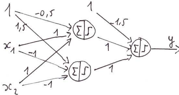
FIGURE 9.4 – Perceptron à une couche cachée calculant le « ou exclusif » (XOR). On vérifie que, selon les valeurs de x_1 et x_2 (0 ou 1), la valeur de y en sortie correspond bien à x_1 \text{ XOR } x_2 .
