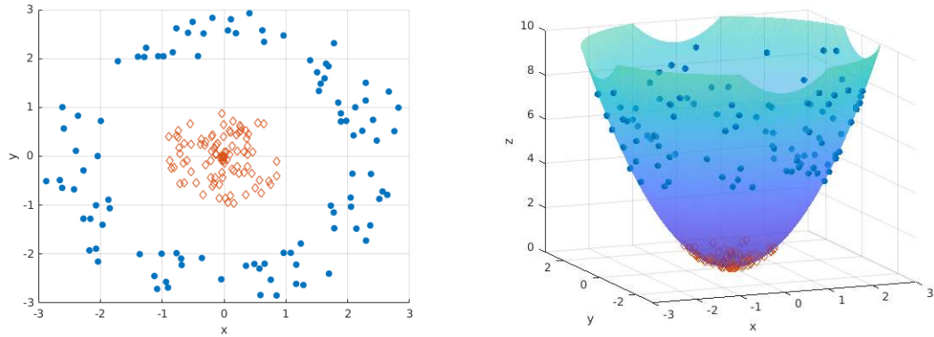
FIGURE 8.4 – Exemple de plongement de points de \mathbb{R}^2 dans \mathbb{R}^3 . Le plongement consiste à projeter les points du plan sur un paraboloïde de révolution de \mathbb{R}^3 . Sur le paraboloïde dans \mathbb{R}^3 les deux classes sont linéairement séparables, ce qui n'était pas le cas dans \mathbb{R}^2 .
