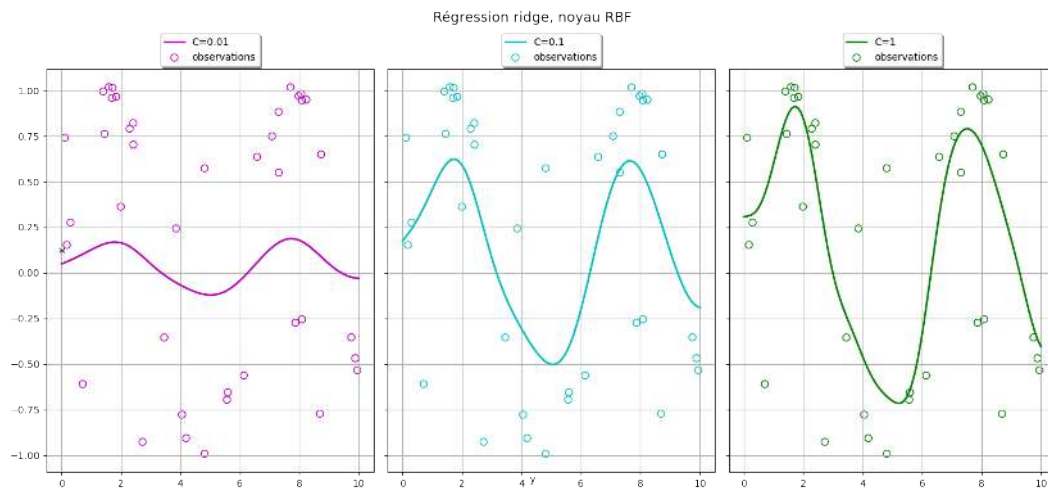
FIGURE 8.10 – Régression ridge à noyau RBF. Plus C est grand, plus les écarts sont pénalisés et plus la courbe de régression s'approche des observations. Un C trop faible implique un sous-apprentissage, un C trop élevé un sur-apprentissage. À comparer à la figure 8.9.
