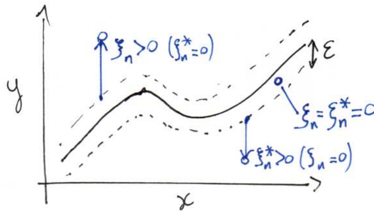
FIGURE 8.8 – Valeurs possibles pour les variables d'écart selon la position relative des observations et de la courbe de régression optimale. Cette représentation anticipe un peu la discussion et l'introduction du noyau pour rendre la prédiction non-linéaire. Trois cas sont possibles à l'optimum du problème de minimisation sous-contraainte définissant la SVR : soit l'observation est dans le \epsilon -tunnel et dans ce cas \xi_n = \xi_n^* = 0 , soit l'observation est « au-dessus » et \xi_n > 0 , \xi_n^* = 0 , soit l'observation est « en-dessous » et \xi_n^* > 0 , \xi_n = 0 .
