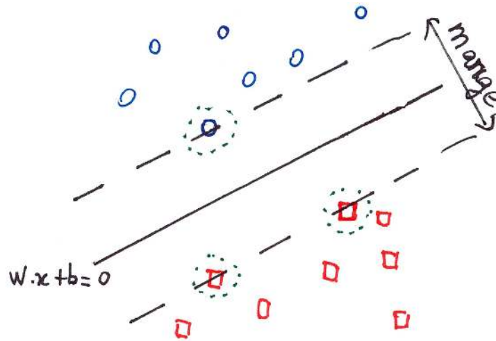
FIGURE 8.1 – Discrimination entre deux classes : marge d'une droite séparatrice d'équation \mathbf{w} \cdot \mathbf{x} + b = 0 et vecteurs supports entourés.
