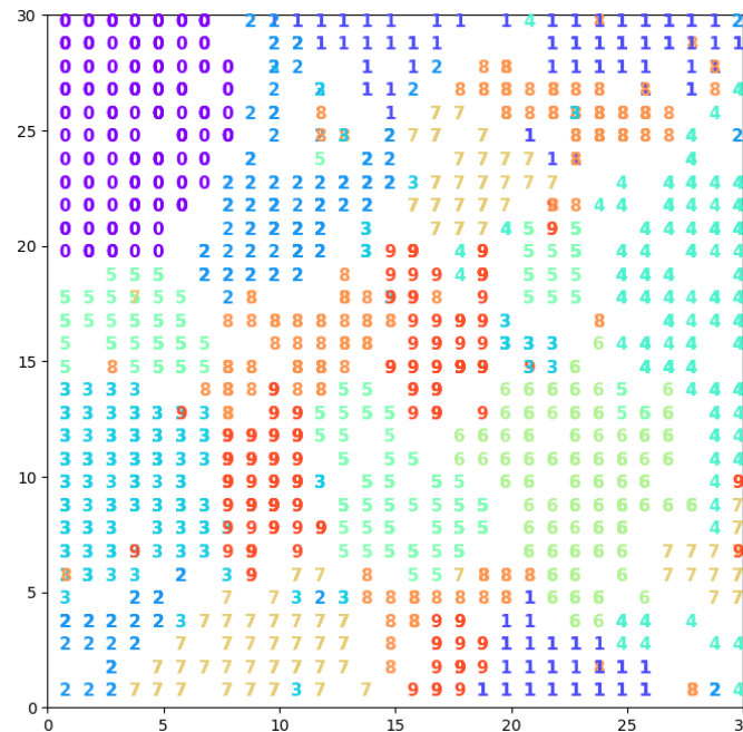
FIGURE 3.7 – On considère un ensemble d'images de tailles 8 \times 8 pixels (l'espace des observations est donc \mathbb{R}^{64} ) et une carte auto-organisatrice planaire rectangulaire de 30 \times 30 nœuds. En chaque nœud un prototype m_k est déterminé par l'algorithme d'apprentissage. La figure montre la superposition des classes affectées à chaque nœud après apprentissage : avec la notation du texte, la classe de chaque observation x_i est affichée en position k^*(i) . On voit que l'essentiel des nœuds ne correspond qu'à des observations x_i d'une seule classe (un seul chiffre apparaît). Certains nœuds n'ont été associés à aucune observation d'apprentissage et forment une « frontière » entre groupes d'observations homogènes. Cette représentation permet une visualisation de l'espace des observations cohérente avec les classes attendues (qui, rappelons-le, sont inconnues). Source et code Python : https://github.com/JustGlowing/minisom/blob/master/examples/HandwrittenDigits.ipynb
